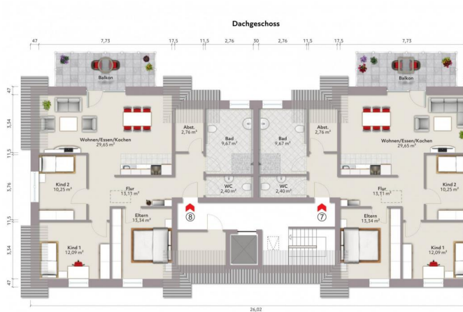
Dachgeschoss Wohneinheiten 7 / 8
