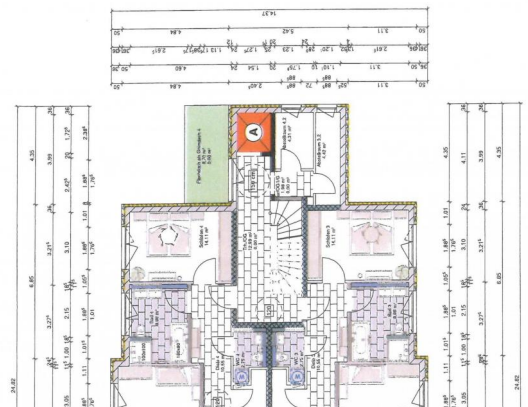
GR 1. Obergeschoss
